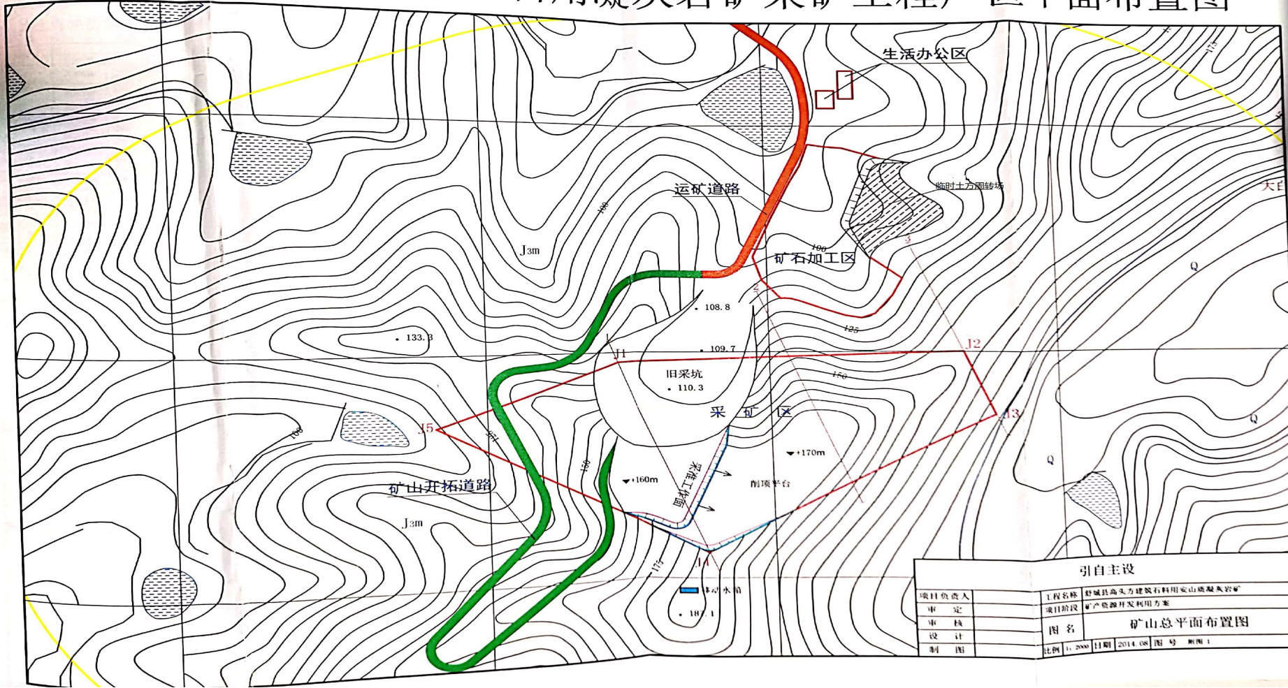
附图1 高头方建筑石料用凝灰岩矿采矿工程厂区平面布置图
