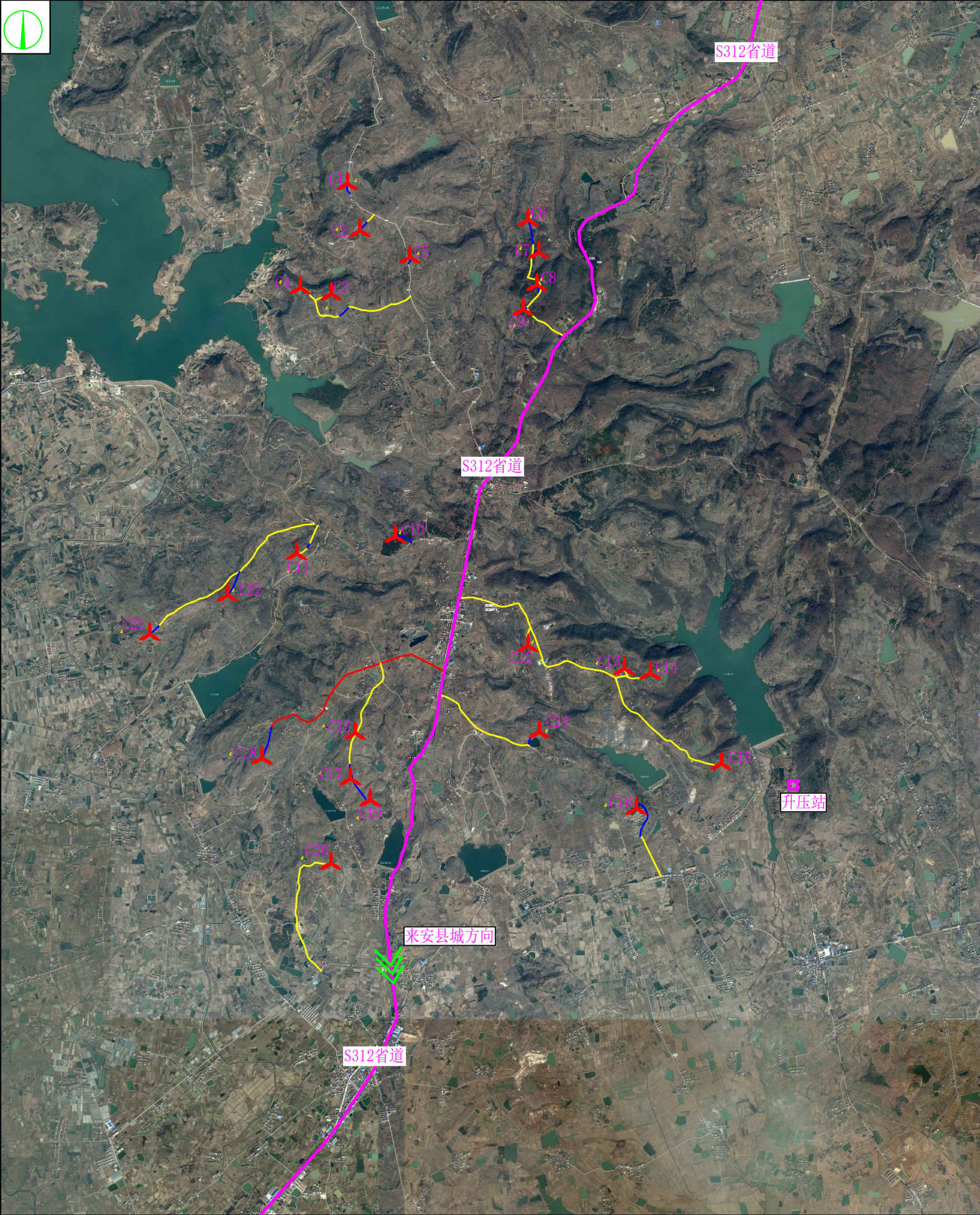
大唐来安张山48兆瓦风电项目-总平面布置图
