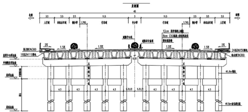
图 1-3 美和路桥梁标准横断面图
