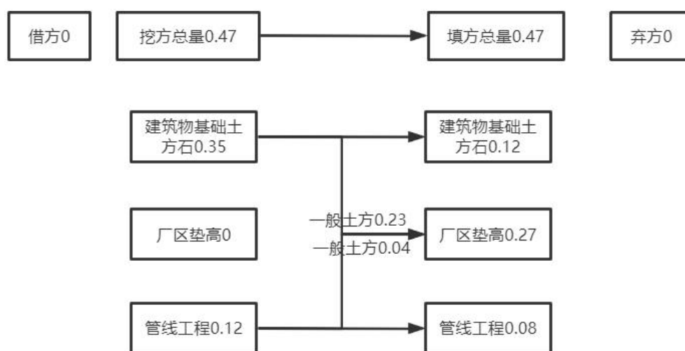
图 1.8-1 项目土石方平衡流向图 单位万 \text{m}^3
