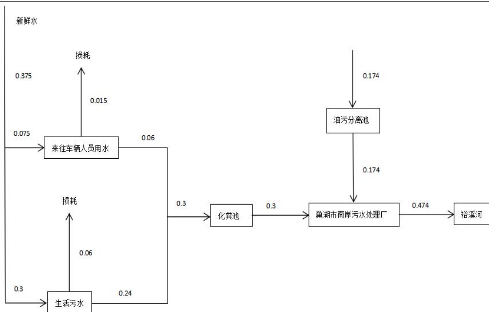
图 2.2-5 项目水平衡图
