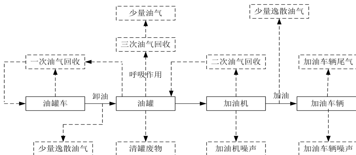
图 2.2-2 汽油加油工艺流程图及产污环节
