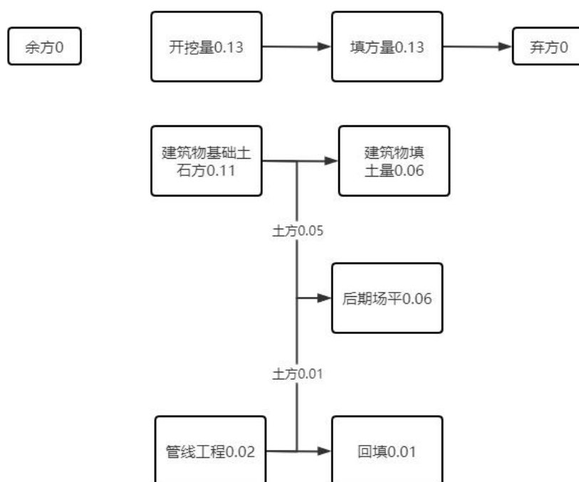
图 1.8-1 项目土石方平衡流向图 单位万 m 3
