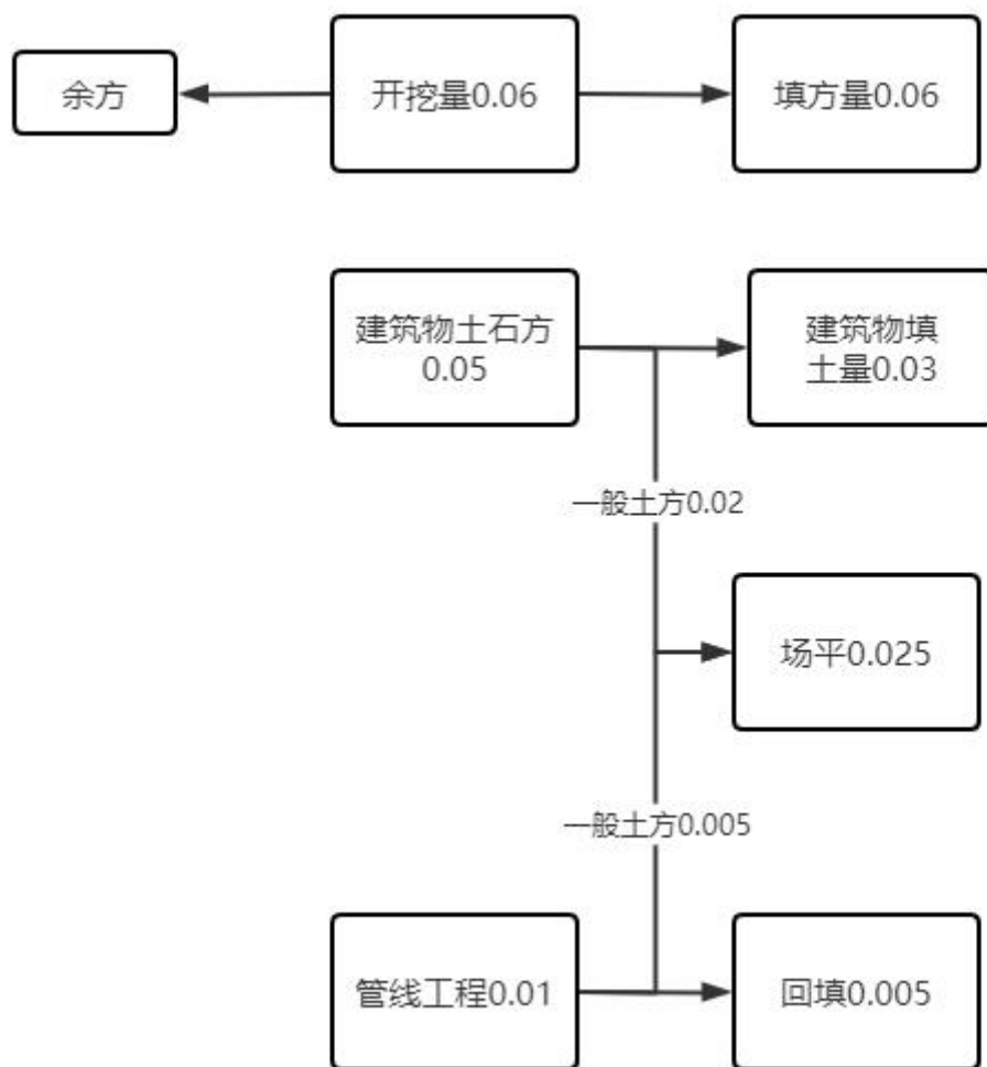
图 1.8-1 项目土石方平衡流向图 单位万 m 3
