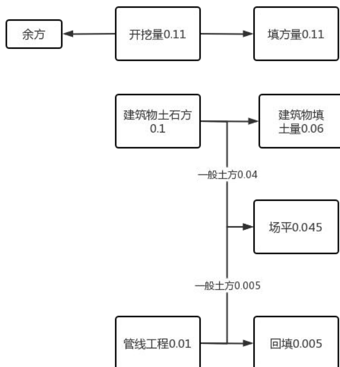
图 1.8-1 项目土石方平衡流向图 单位万 \text{m}^3
