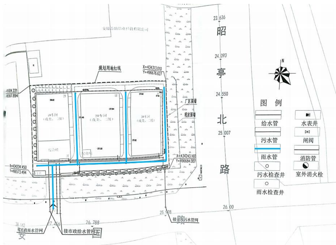
图 1.5-3 本项目雨水管网分布示意图
