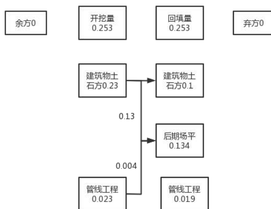
图 1.8-1 项目土石方平衡流向图 单位万 m 3
