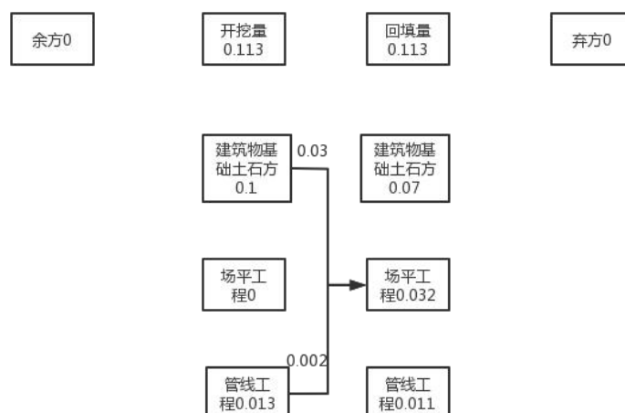
图 1.8-2 项目预计发生土石方平衡流向图 单位万 m 3
