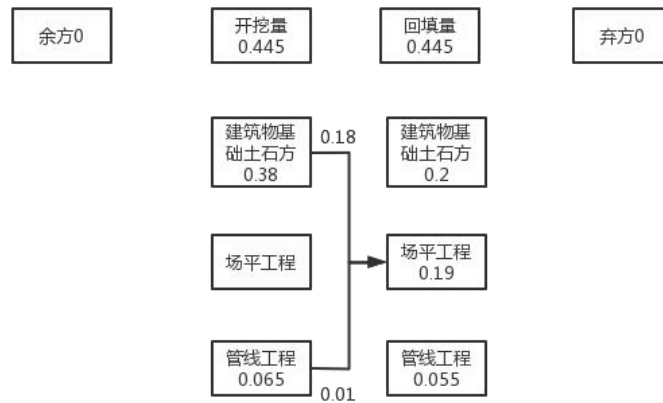
图 1.8-3 项目土石方总体平衡流向图 单位万 m 3
