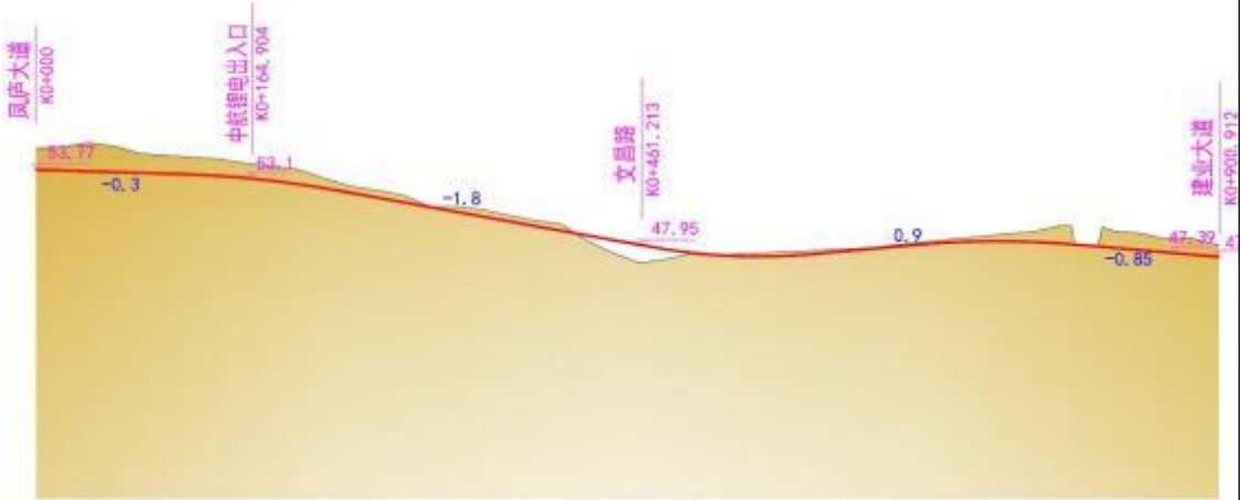
图 4-2 纵断面示意图
