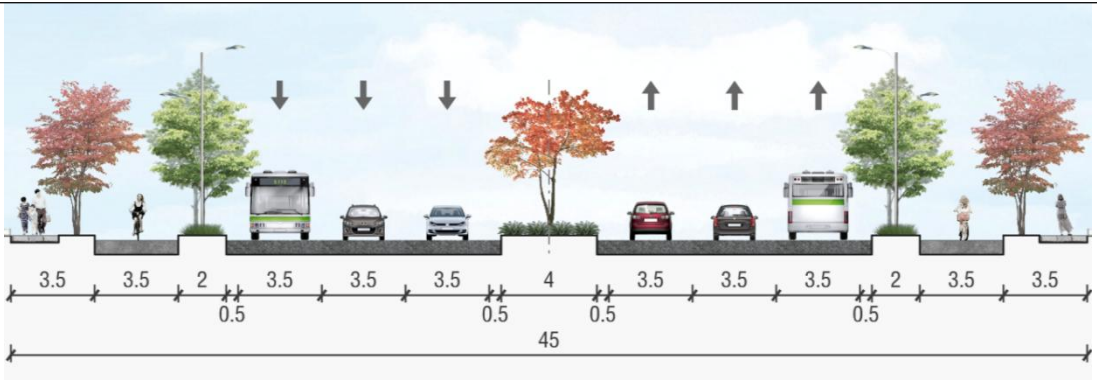
图 4-1 道路标准横断面图
