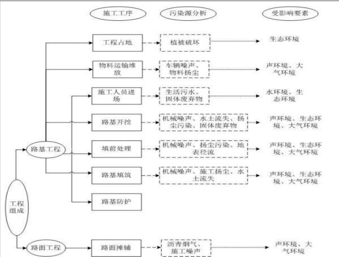
图 4-4 施工工艺流程图
